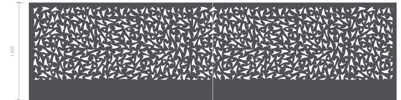
Vorgesetzte Brüstung
