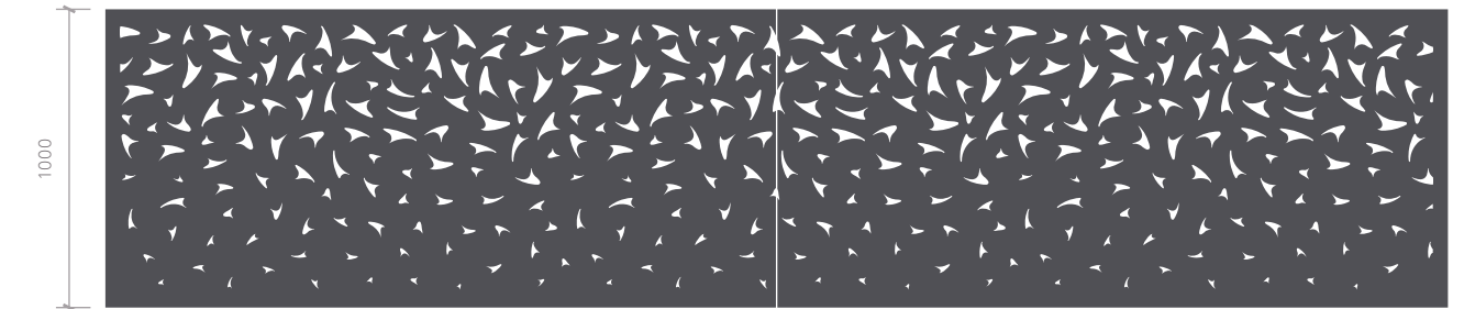
Aufgesetzte Brüstung
